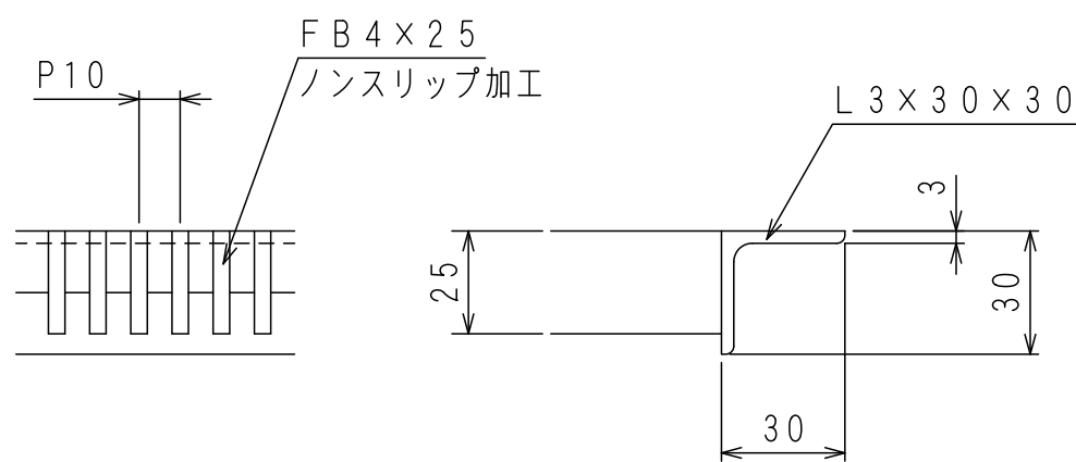
断面詳細 S=1:2
