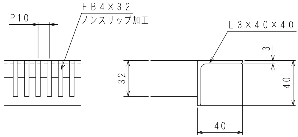
断面詳細 S=1:2
