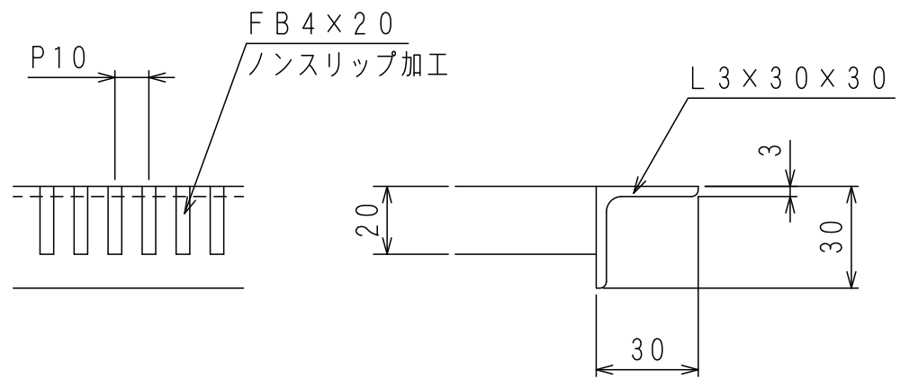
断面詳細 S=1:2
