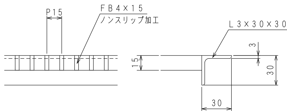
断面詳細 S=1:2
