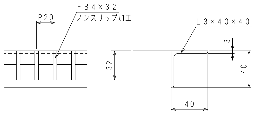
断面詳細 S=1:2
